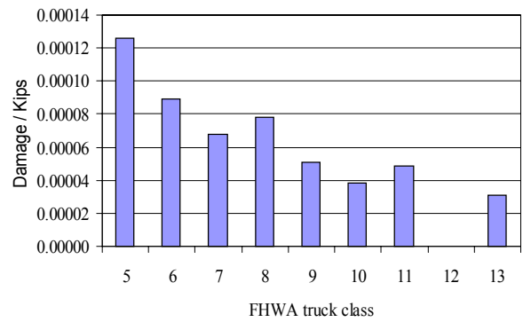
(d) Normalized damage vs. FHWA truck classes
